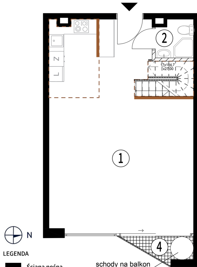
PLAN APARTAMENTU
